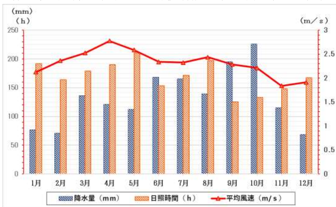
降水量、日照時間及び平均風速の月別推移（平成26年から令和3年までの平均）
